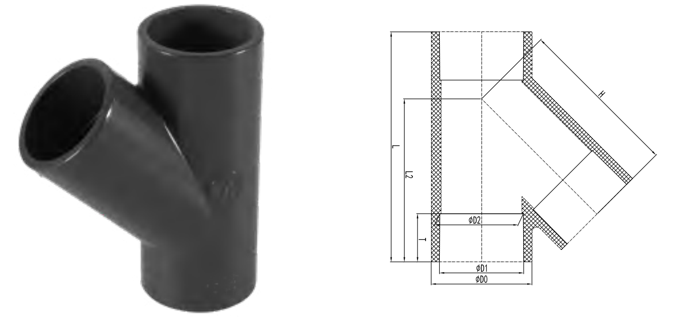
产品参数（国标 GB/T 4219.2） SPECIFICATIONS(DIN,ISO,GB/T)
