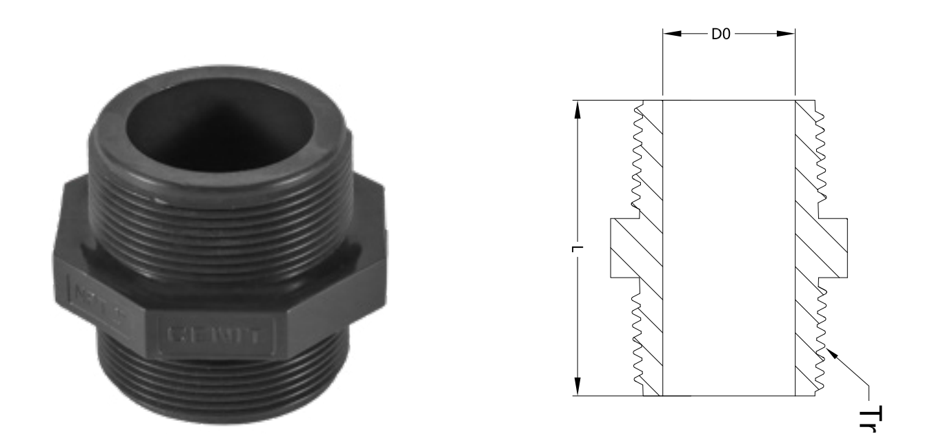
产品参数（美标 SCH80） SPECIFICATIONS(ASTM D2467 SCH80)
